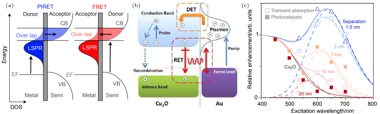
图 3 Au@SiO 2 @Cu 2 O 体系的 PRET/PIRET 增强光催化 [3, 13] (a) PRET/PIRET 和 FRET 示意图, PIRET 是指 Au 等离激元吸收能量转移至 Cu 2 O 中, 而 FRET 则是 Cu 2 O 吸收能量转移至 Au 中; (b) SiO 2 层可以阻止等离激元热电子转移过程 (DET); (c) 相对增强因子随激发波长的变化关系
