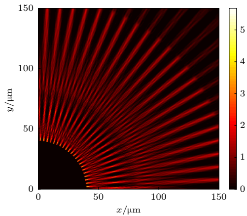
图 2 Lumerical 模拟结果 (光栅内的光场已去除)
