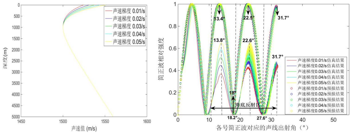
(彩色印刷) 图 8 声速梯度变化时声场角谱域分布 WKBZ 仿真结果与理论预报结果比较 (a)不同跃变层声速梯度下声速剖面; (b)结果比较
