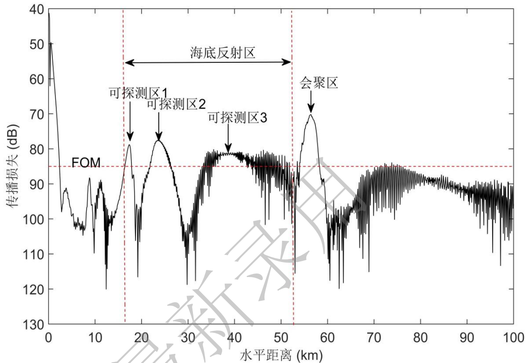
图 2 典型深海 Munk 声道下接收深度固定时声传播损失随距离的变化
