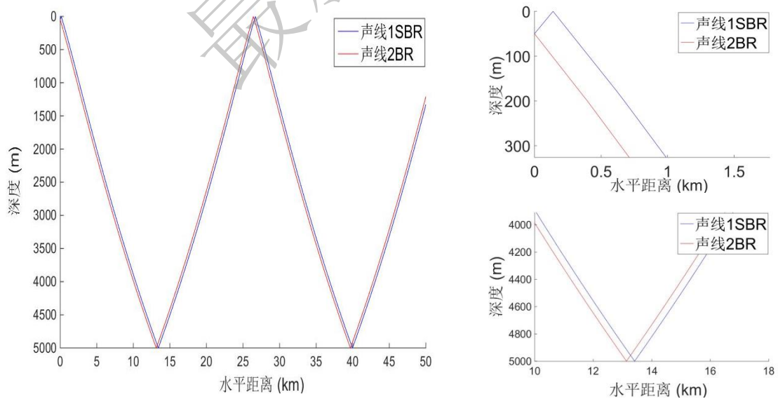
(彩色印刷) 图 5 角谱域上 20^\circ 掠射角对应的两种声线示意图
