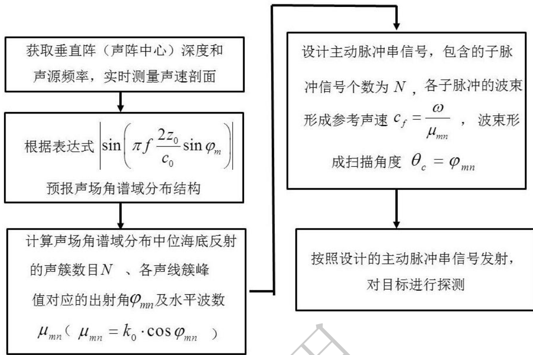
图 11 基于声场角谱域分布结构的主动声纳发射脉冲串信号设计
