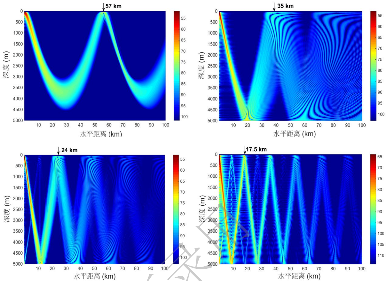
(彩色印刷) 图4 不同简正波(声线)簇形成的声场 (a) 1至120阶简正波(出射角 0^{\circ} - 9.5^{\circ} 的声线)叠加声场; (b)121至216阶简正波(出射角 9.5^{\circ} - 18.2^{\circ} 的声线)叠加声场; (c)217至314阶简正波(出射角 18.2^{\circ} - 27.6^{\circ} 声线)叠加声场; (d)315至354阶简正波(出射角 27.6^{\circ} - 31.7^{\circ} 声线)叠加声场
