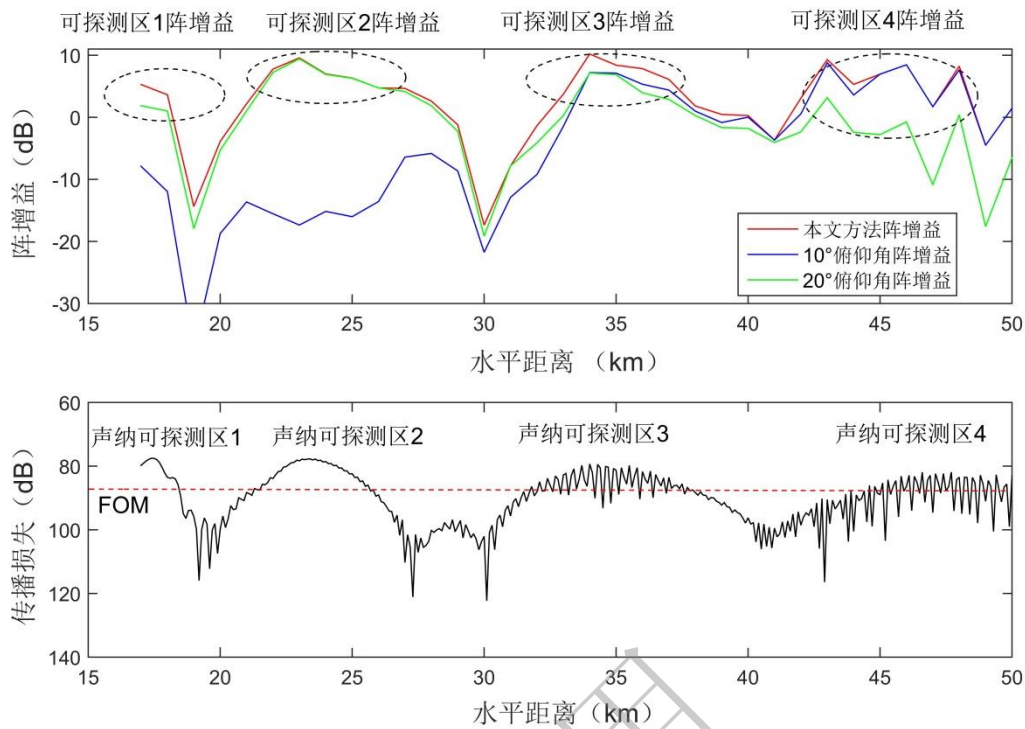
(彩色印刷) 图 13 本文方法和随机设置方法阵增益比较图
