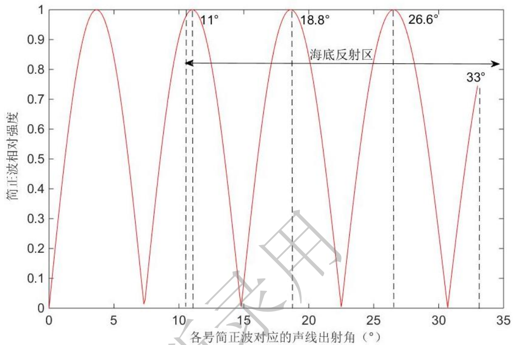
图 12 声场角谱域分布结构
