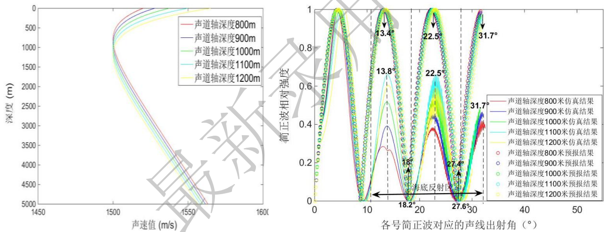
(彩色印刷) 图 9 声道轴深度变化时声场角谱域分布 WKBZ 仿真结果与理论预报结果比较 (a)不同声道轴深度下声速剖面; (b)结果比较
