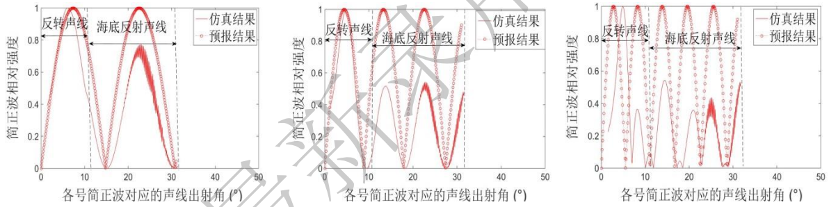
图 7 声源深度变化时声场角谱域分布 WKBZ 仿真结果与理论预报结果比较（声源频率 100Hz） (a) 声源深度 30m; (b) 声源深度 50m; (c) 声源深度 80m
