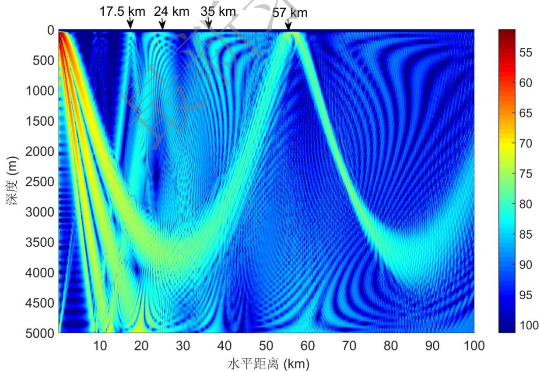
(彩色印刷) 图 1 典型深海 Munk 声道下声传播损失随距离和接收深度变化情况
