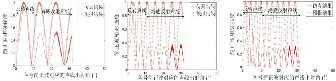
图 6 声源频率变化时声场角谱域分布 WKBZ 仿真结果与理论预报结果比较（声源深度 50m） (a) 声源频率 100Hz; (b) 声源频率 200Hz; (c) 声源频率 300Hz
