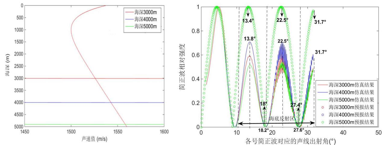
(彩色印刷) 图 10 海深变化时声场角谱域分布 WKBZ 仿真结果与理论预报结果比较
