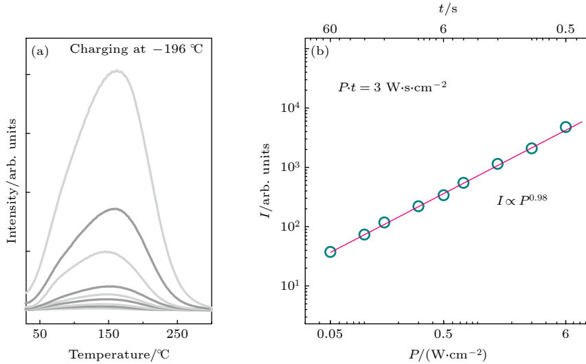
图 4 (a) 通过固定辐照剂量 ( 3 \text{ W s cm}^{-2} ) 的上转换充能后, \text{LaMgGa}_{11}\text{O}_{19}:\text{Mn}^{2+} 材料的热释光谱 ( 450 \text{ nm} 激光的辐照功率密度分别为: 0.05, 0.1, 0.15, 0.3, 0.5, 0.75, 1.5, 3, 6 \text{ W cm}^{-2} ); (b) 热释光积分强度 I 随辐照功率密度 P 的变化及 I-P 函数拟合
