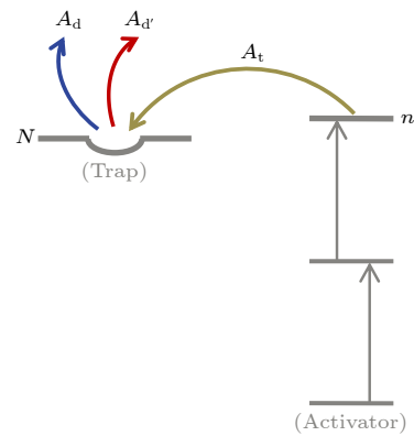
图 5 考虑了光激励排空和其他激励排空影响的上转换充能动力学示意图
