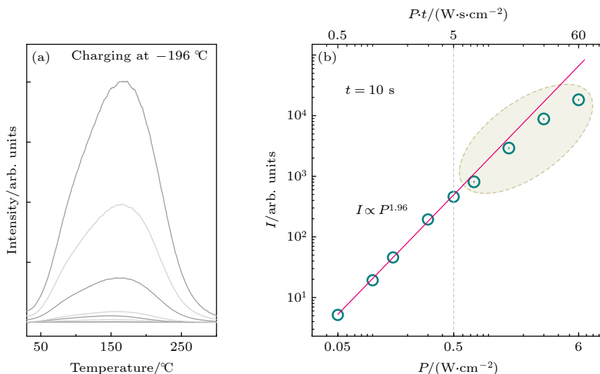
图 3 (a) 通过固定辐照时长 (10 s) 的上转换充能后, \text{LaMgGa}_{11}\text{O}_{19}:\text{Mn}^{2+} 材料的热释光谱 (450 nm 激光的辐照功率密度分别为 0.05, 0.1, 0.15, 0.3, 0.5, 0.75, 1.5, 3, 6 \text{ W}\cdot\text{cm}^{-2} ); (b) 热释光积分强度 I 随辐照功率密度 P 的变化及 I - P 函数拟合
