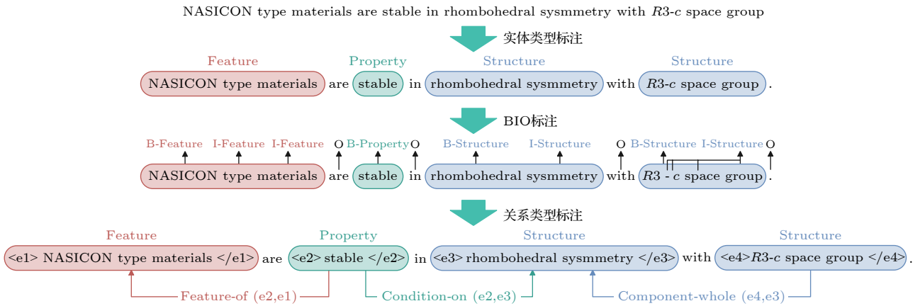
图 3 实体关系标注流程示意图
