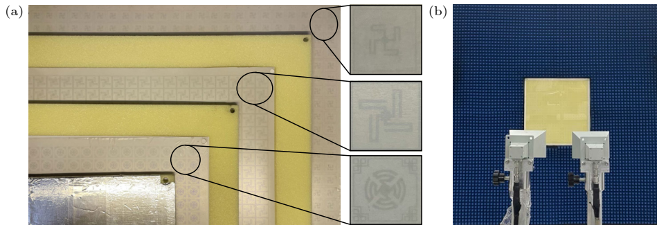
图 12 (a) 加工样件; (b) 实验测试系统 Fig. 12. (a) Fabricated prototype; (b) the experimental setup.
