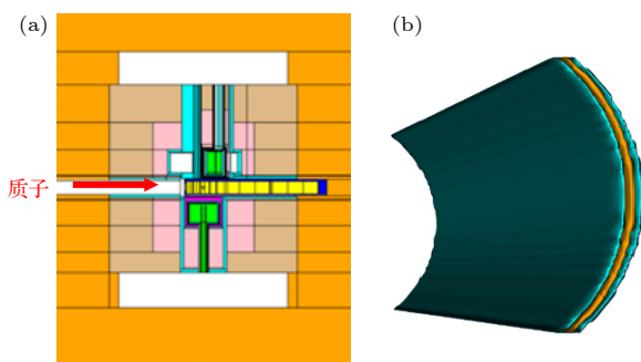
图 5 靶站几何模型 (a) TMR 系统 y - z 轴截面图, 其中 +y 为质子入射方向; (b) 质子束窗
