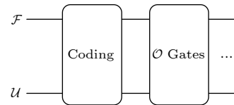
图 5 量子资源理论框架下的计算模型. 第 I 类模型主要是针对输入端, 即信息不同表示形式; 第 II 类模型主要是针对编码后的逻辑操作的形式
