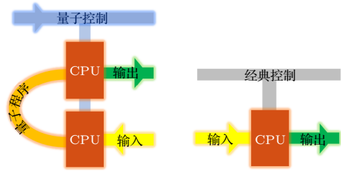
图 8 量子冯·诺依曼架构示意图 (左) 与量子线路模型 (右). 对比来看, 在通常的线路模型中不考虑量子的控制单元和量子的程序存储
