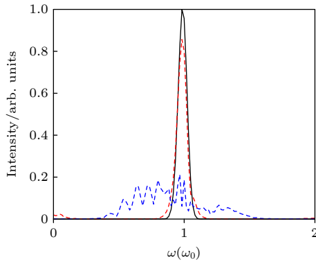
图 5 小能量长脉冲激光在莫尔晶格与抛物型通道中的导引效果对比. 黑色实线表示 t = 0 时刻的入射光光谱, 红色虚线与蓝色虚线表示激光分别在莫尔晶格与抛物型通道中传播 d = 800\lambda_0 的光谱
