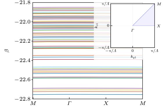
图 2 莫尔晶格的近似能带
