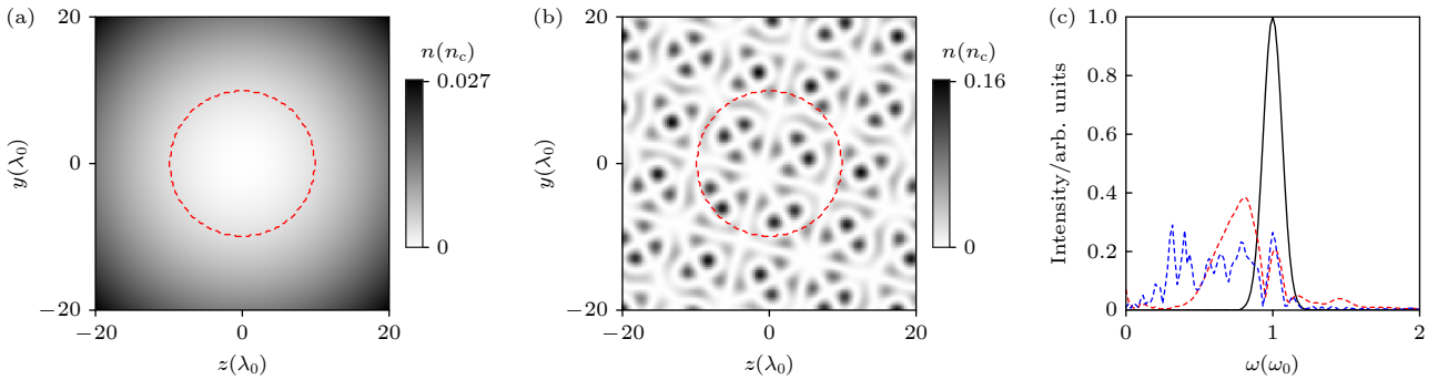
图4 莫尔晶格与抛物型通道导引效果对比(其中红色虚线圆圈表示距离中心 r=10\lambda_0 的区域) (a) 抛物型通道横向密度分布; (b) 莫尔晶格横向密度分布; (c) 黑色实线表示 t=0 时刻的入射光光谱,红色虚线与蓝色虚线表示激光分别在莫尔晶格与抛物型通道中传播 d=800\lambda_0 的光谱
